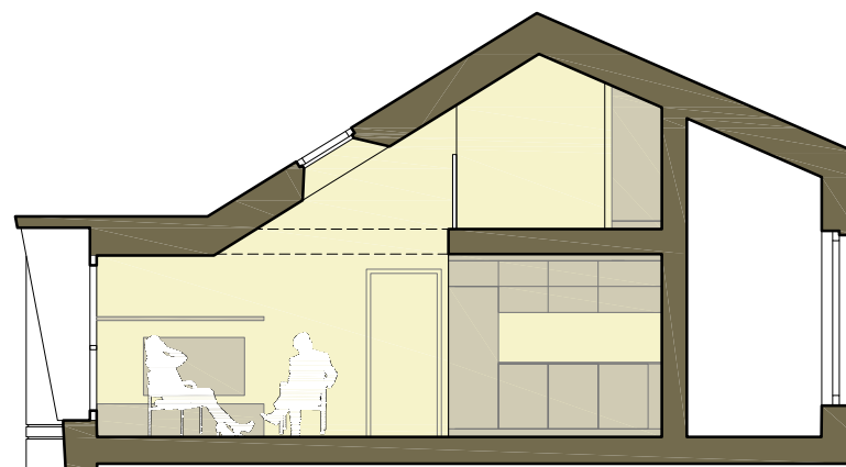
příčný řez
