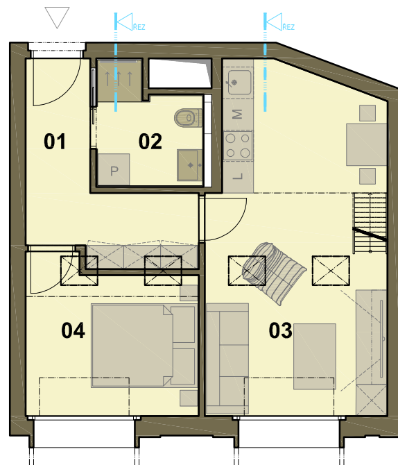
1. patro
